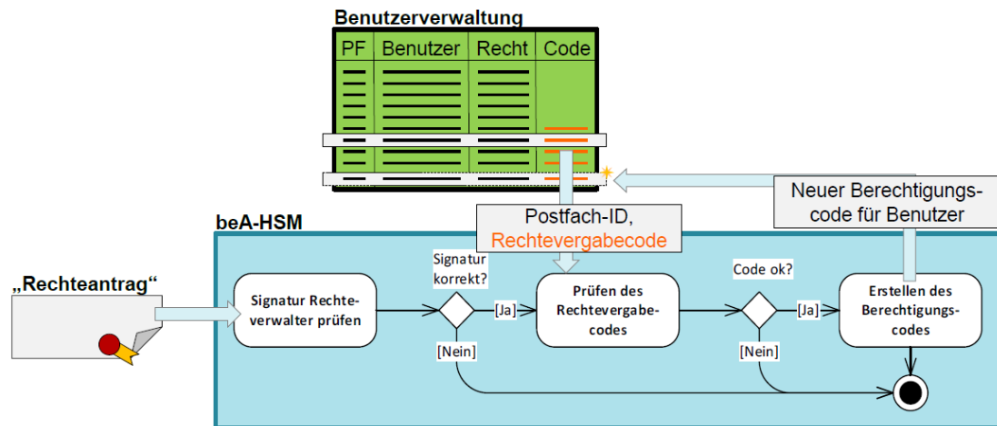
Abbildung 6: Management von Administrations- und Leserechten
